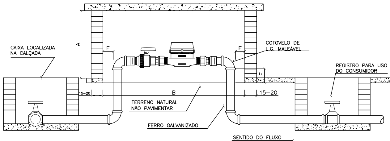
ELEVAÇÃO
